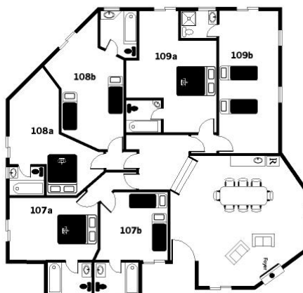
Maisonnettes 107a et 107b - 108a et 108b 109a et 109b
